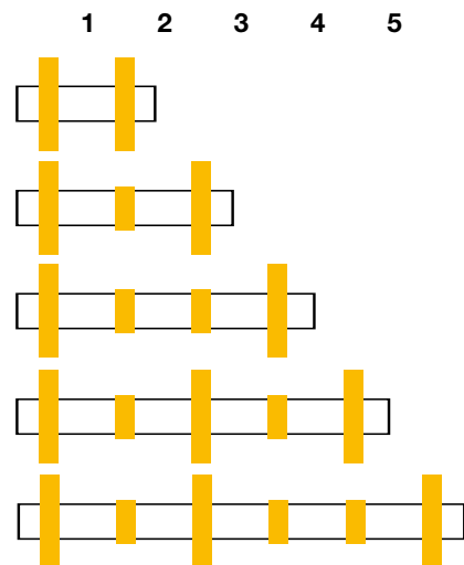
Positions des supports en T lors de l'utilisation de plusieurs unités
